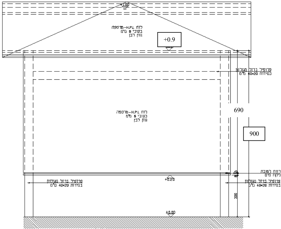
מבט 2 (גב) קני"מ 1:5
