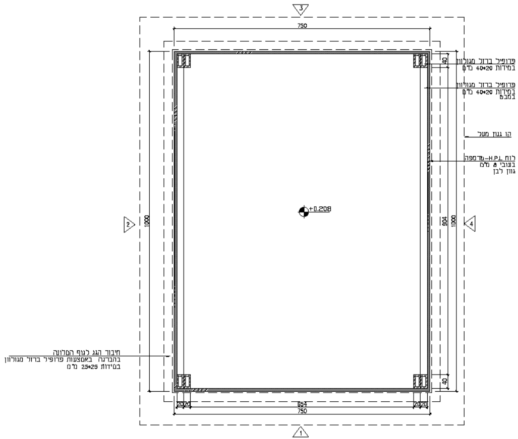
תכנית קני"מ 1:5
